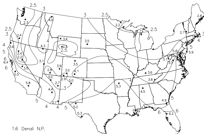
S.2(a) Total light extinction b_{ext} ( \text{Mm}^{-1} )
