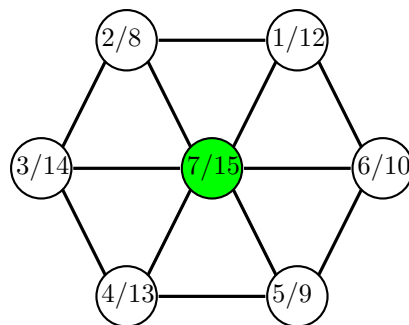
Figura 7.32: Grafo que no es adecuado para el algoritmo goloso
