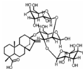
Rebaudioside B
