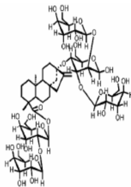
Rebaudioside D
