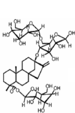
Stevioside
