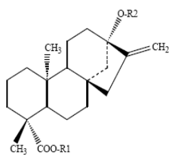
Steviol
