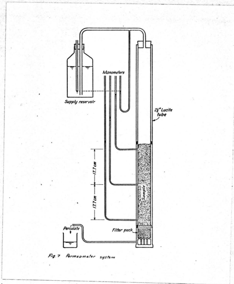
Fig. 7 Permeameter system.
